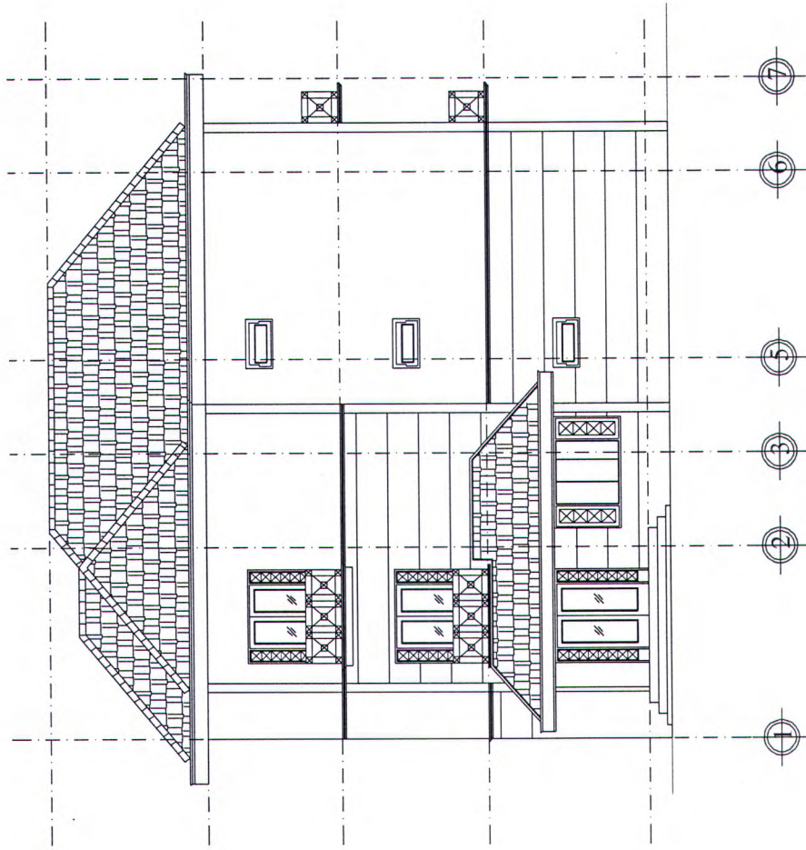
MẶT ĐÚNG 1 - 7 TL : 1/100
