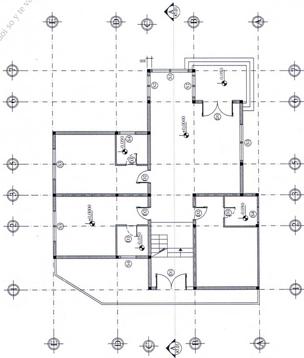
MẶT BẰNG TRỆT TL : 1/100
