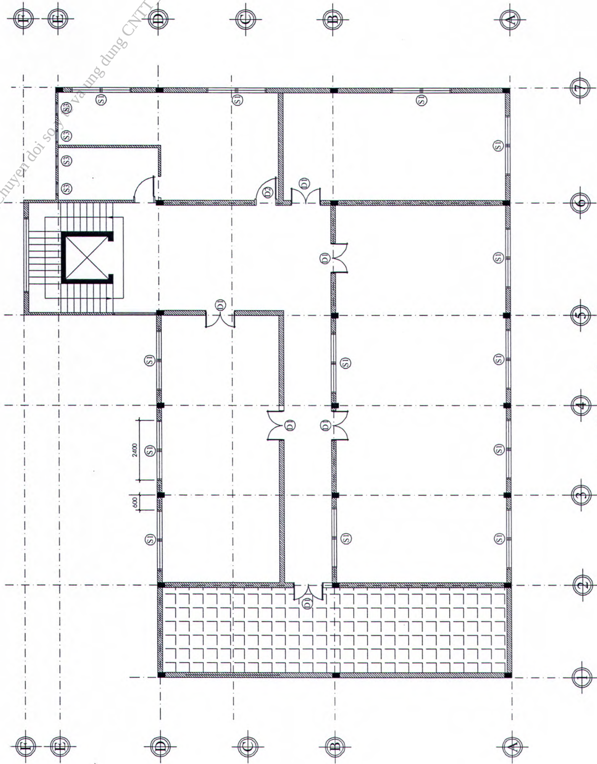
MẶT BẰNG LẦU 2 TL : 1/100
