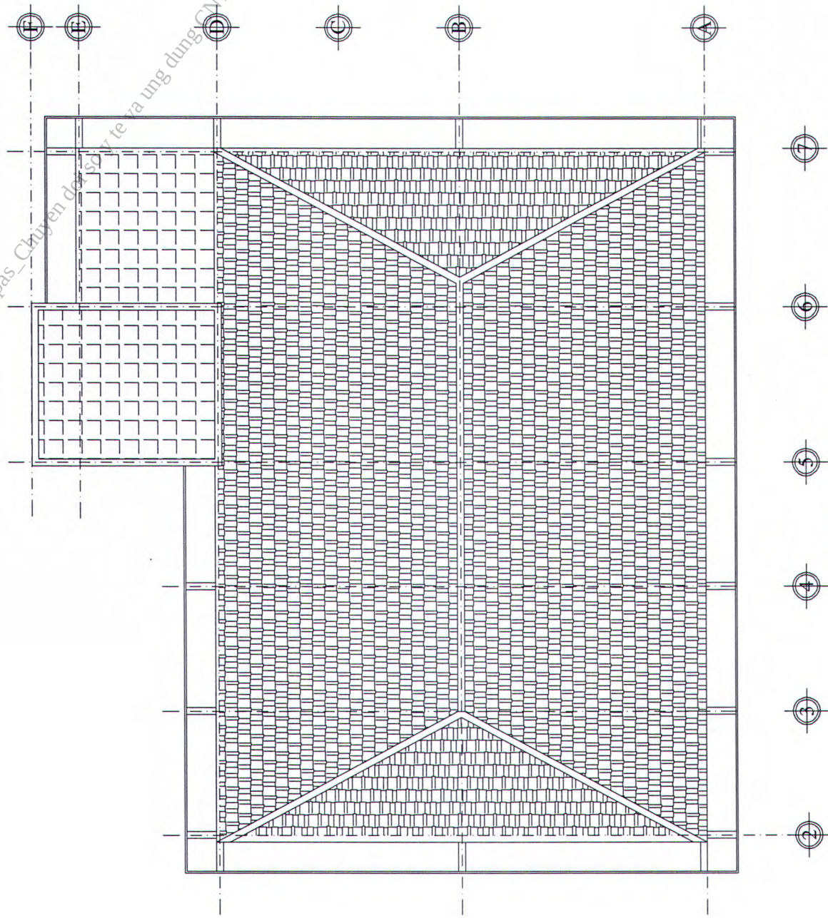
MẶT BỀ MẶT MÁI TL : 1/100
