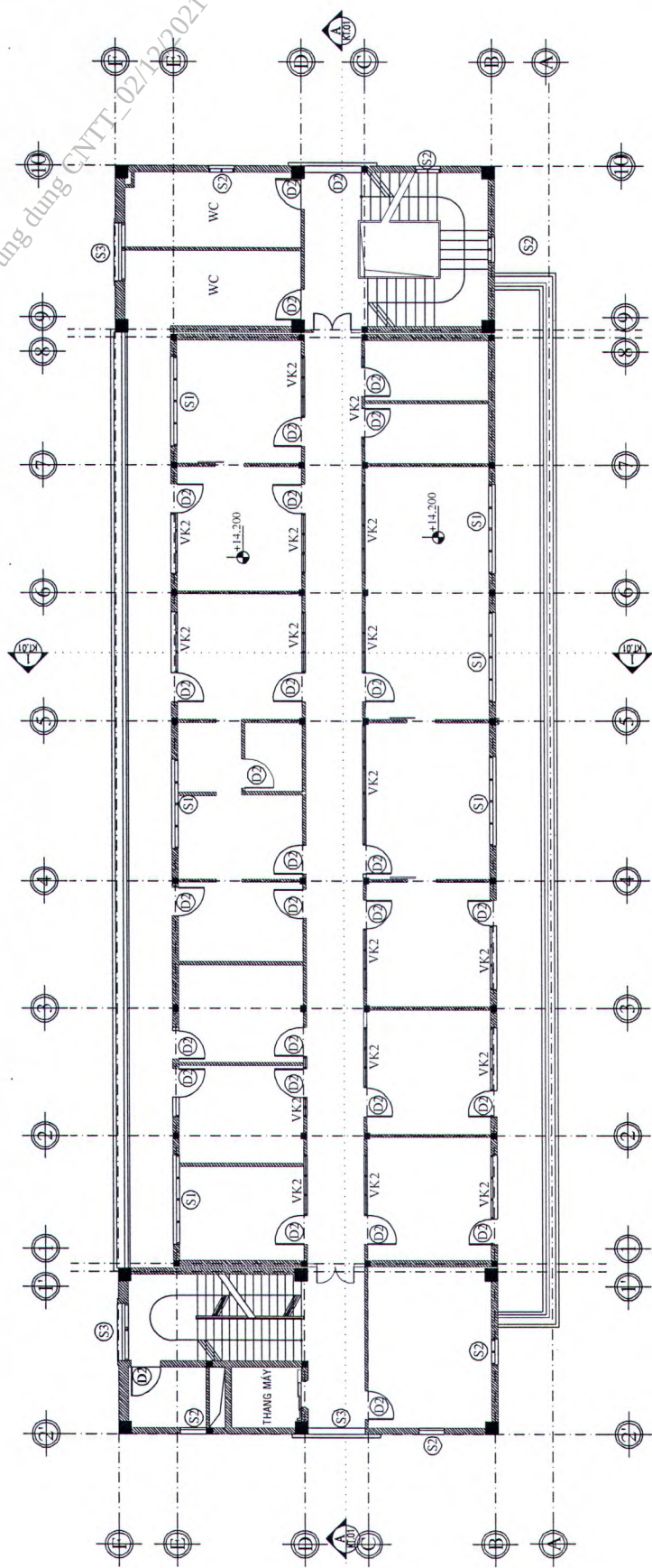
MẶT BẰNG LẦU 4 TL 1/100
