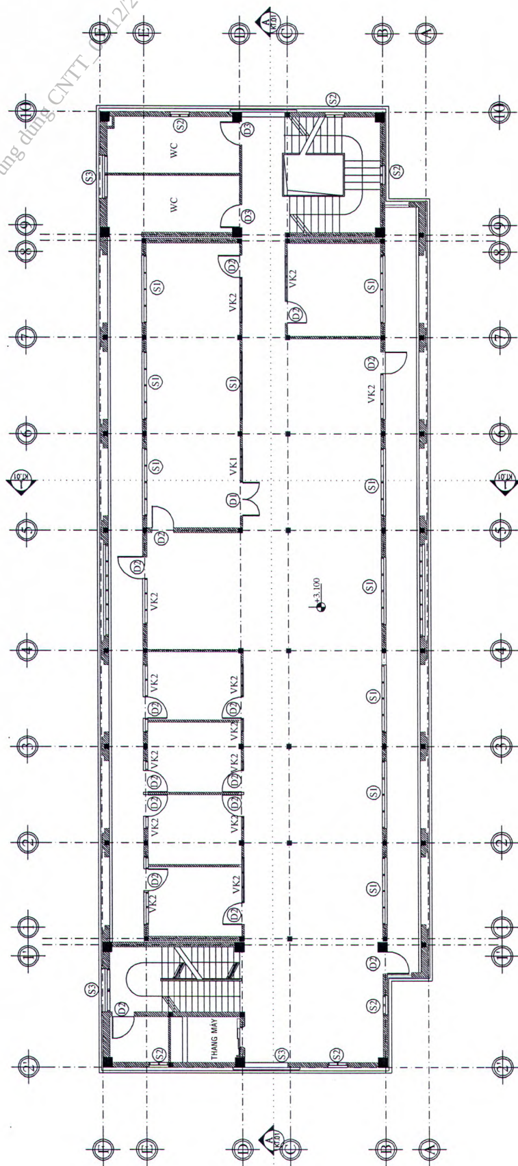
MẶT BẰNG LẦU 1 TL 1/100
