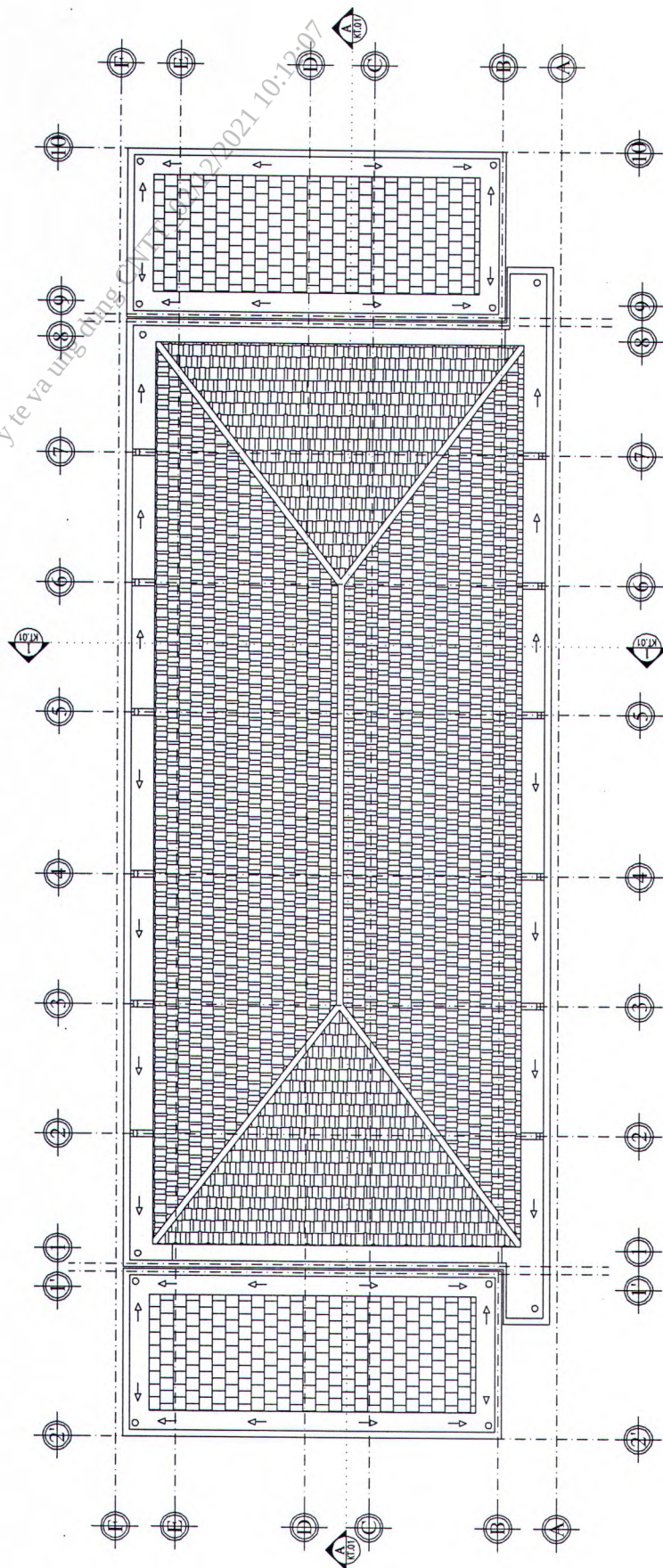
MẶT BỀ MẶT MÁI TL 1/100
